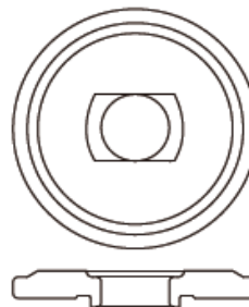
Inner flange 45 (224399-1)
